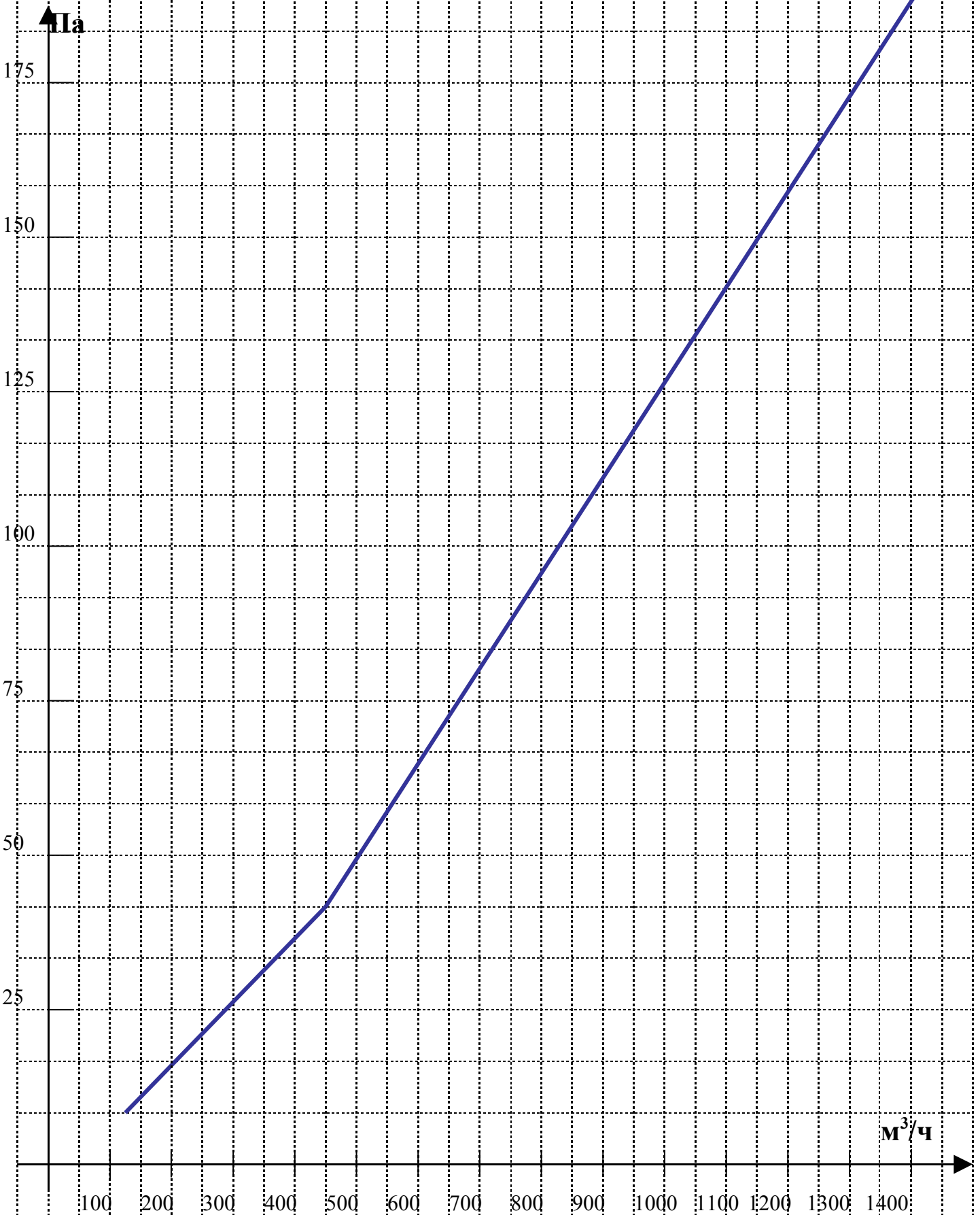
График перепада давления на фильтрующем блоке ФБ-25031
