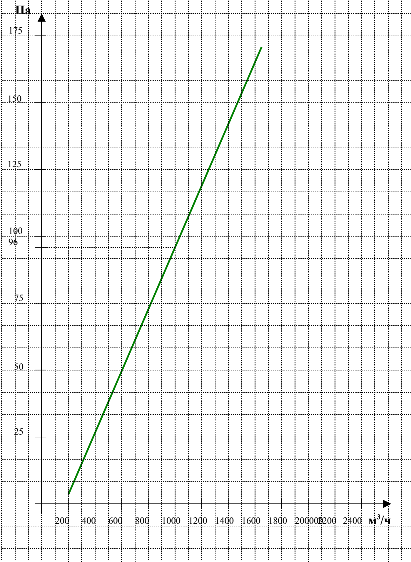
График перепада давления на угольной фильтр-кассете УФ-1-251 (1000 м 3 /ч)
